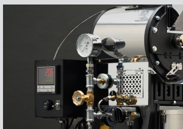
ガス圧力計
