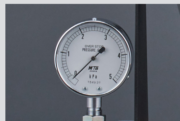
ガス圧力計
